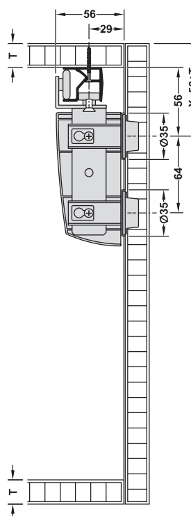
Монтажные размеры
