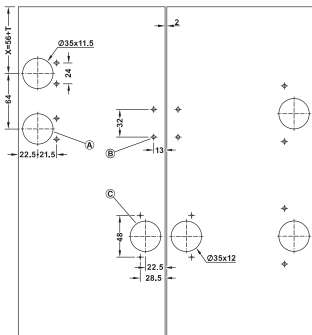
Схема сверления дверного полотна
