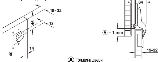
Схема сверления для крепления чашки
