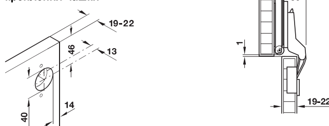
Схема сверления для крепления чашки
