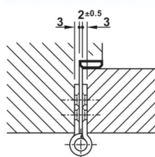
Монтаж петель 926.98.xxx
