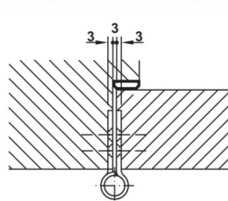
Монтаж петель 926.90.213 и 926.90.290
